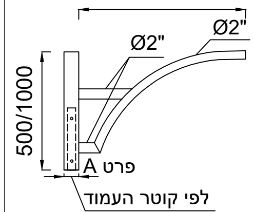
חיבור פנס תפיסה מהצד
