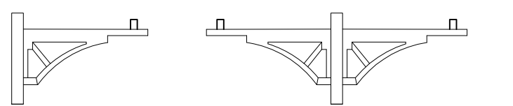
חיבור פנס הלבשה ראש עמוד
